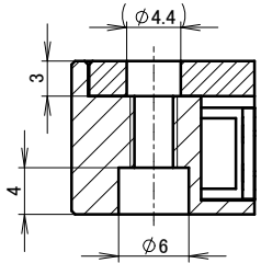
A-A (2 : 1)
