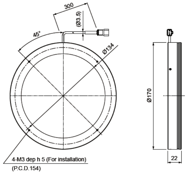
LDR2-170RD2-LA / SW2-LA / BL2-LA / GR2-LA
