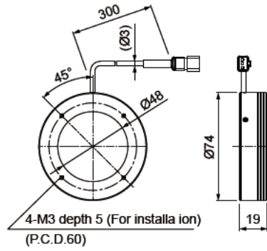
LDR2-74RD2-LA / SW2-LA / BL2-LA / GR2-LA
